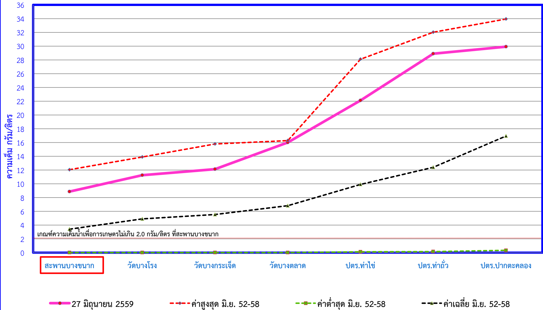
ค่าความเค็มในแม่น้ำบางปะกง วันที่ 27 มิถุนายน พ.ศ. 2559
